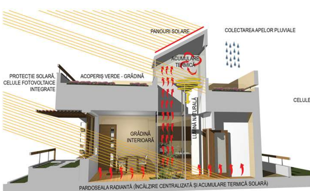
CONCEPTUL BIOCLIMATIC DE FUNCȚIONARE - IARNA
